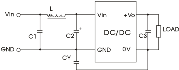
(图 4) EMC 推荐电路
