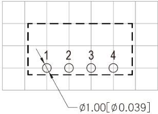
栅格距离: 2.54×2.54mm ( 顶视图 ) 推荐 PCB 封装脚位
